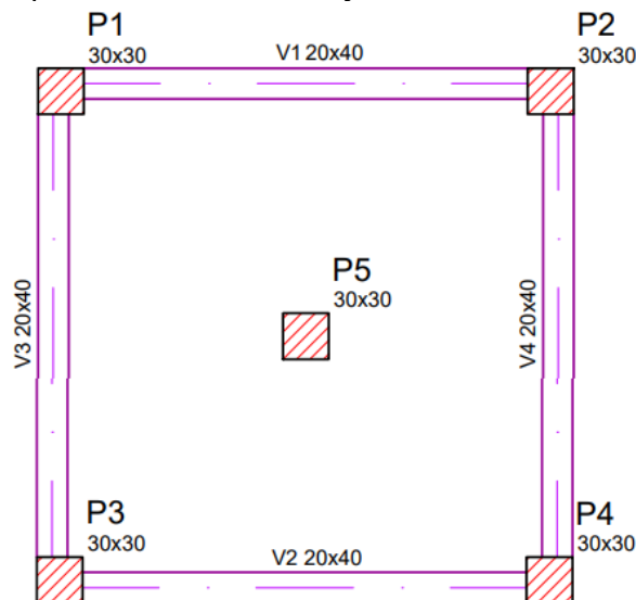
Figura 2: Forma do travamento intermediário
