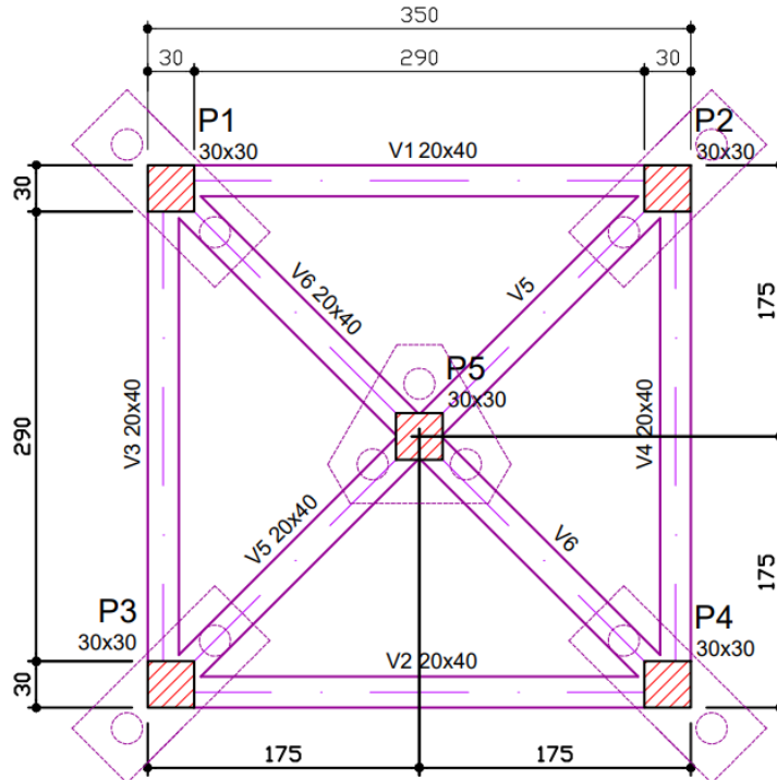
Figura 1: Forma do pavimento base de fundação
