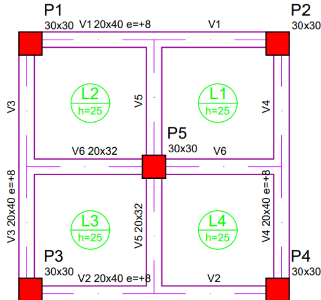
Figura 3: Forma da laje suporte do reservatório
