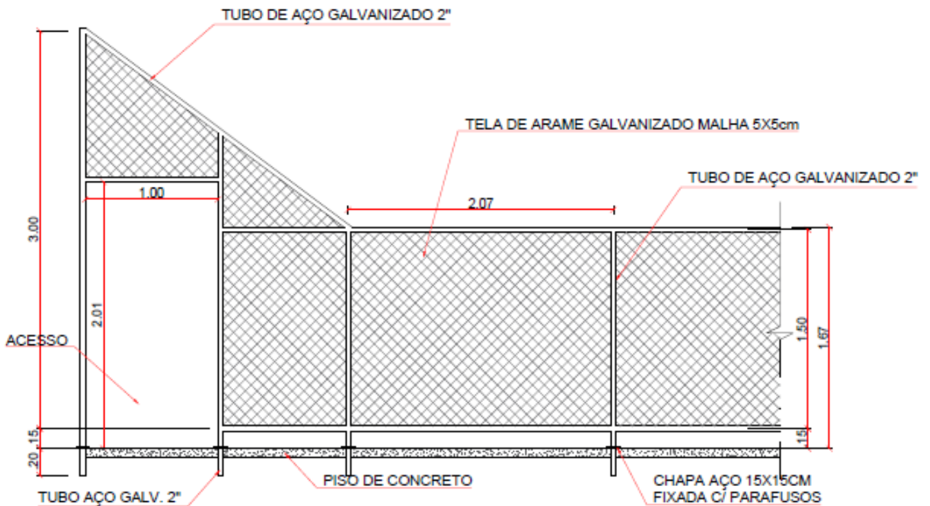
VISTA DO ALAMBRADO (LATERAL) SEM ESCALA
