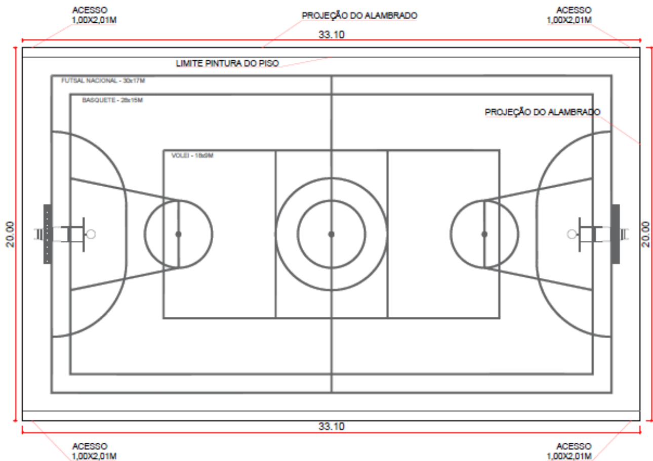
PLANTA BAIXA - ALAMBRADO SEM ESCALA
